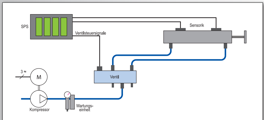
Schematische Darstellung der erforderlichen Komponenten für eine pneumatische Achse
