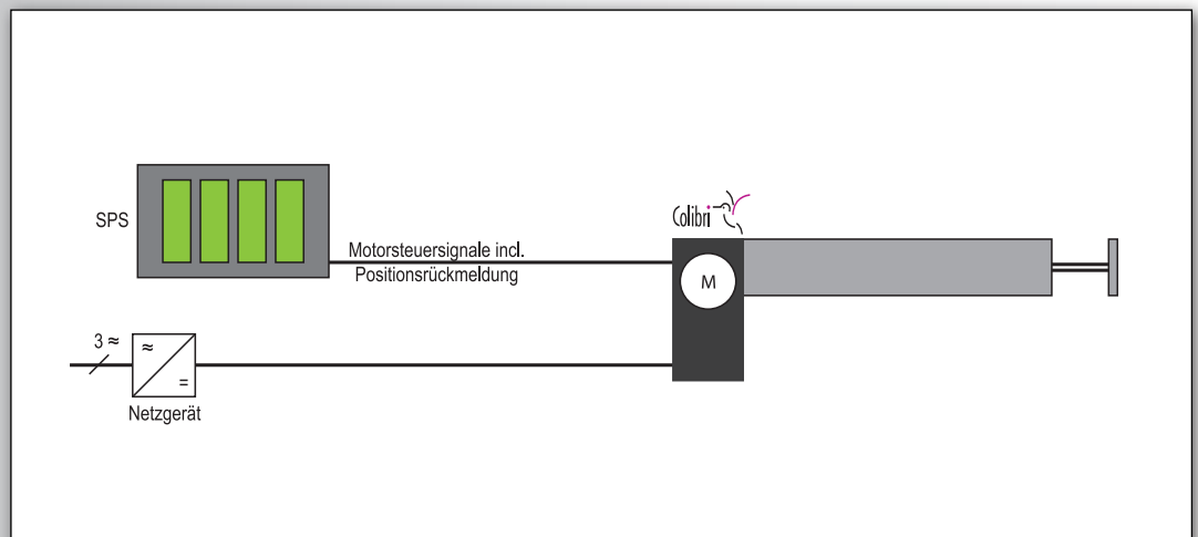
Schematische Darstellung der erforderlichen Komponenten für eine Colibri - Achse
