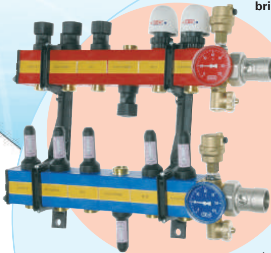
SBK-Heizkreisverteiler 3000
