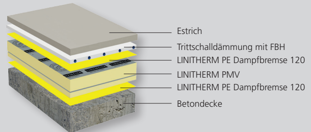
Wärmedämmung unter Estrich mit Fußbodenheizung
