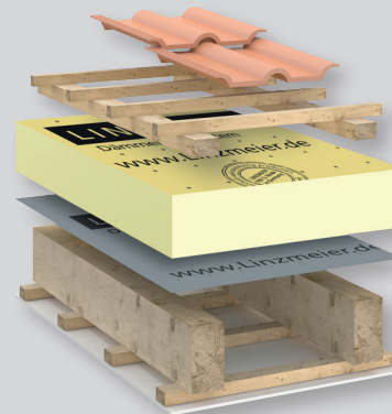
Aufsparrendämmung LINITHERM PAL N+F mit verkleideten Sparren und raumseitiger Bekleidung
