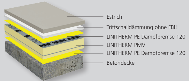
Wärmedämmung unter Estrich ohne Fußbodenheizung
