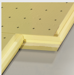
LINITHERM PAL N+F mit speziellem Stecksystem und Klemm-Press-Verbindung
