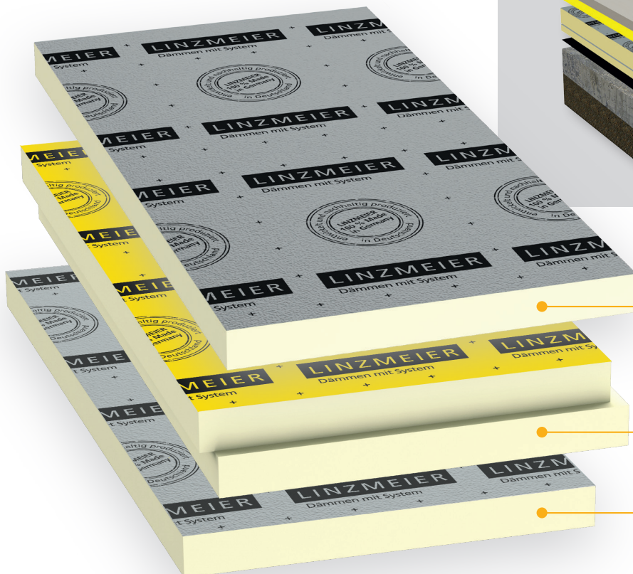
Wärmedämmung unter Estrich gegen Erdreich
