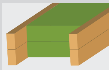
280 mm dick: Mineralfaser \lambda_B 0,035 W/(mK) zwischen den Sparren
