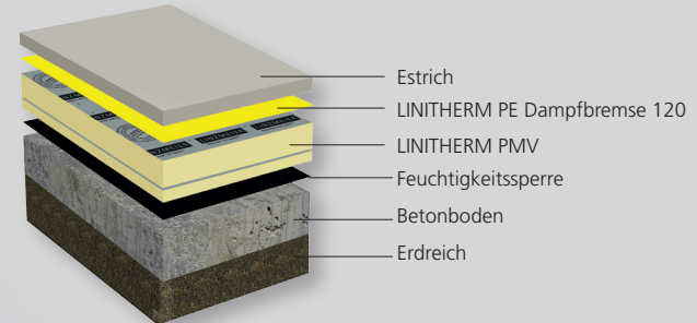
Wärmedämmung unter Estrich gegen Erdreich
