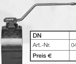
Kompaktkugelhahn INTEC 112 FS (voller Durchgang TA-Luft) Gehäuse: Edelstahl (1.4571 / 1.4541) / Kugel: Edelstahl / Dichtungen: PTFE
