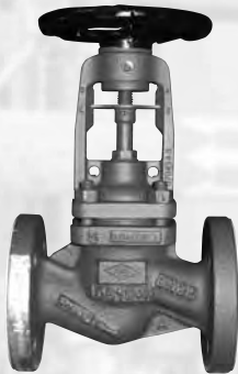
ARI-Faltenbalgventil Supra I Stahlguß, doppelwandiger Faltenbalg verschweißt, Kantensitzkegel einteilige Spindel (TA-Luft-Zulassung)
