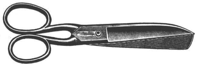
Art. 620 Materialscherer , solide kräftige Ausführung aus blankem Stahl, für Leder und andere Stoffe Normallänge ca. 205 mm .....
