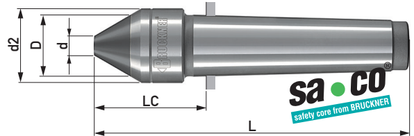
Form R großer Hartmetallring bis \varnothing 100 \text{ mm}
