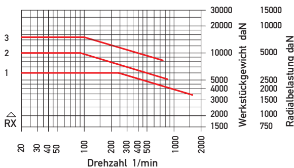
Radial – Typ MZ, AMZ, MZR
