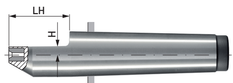
Form HB, abgeflacht *Rundheitstoleranz \square \leq 1 \mu\text{m}
