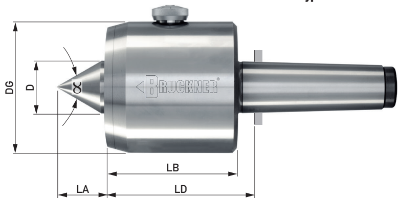
Typ MZ
