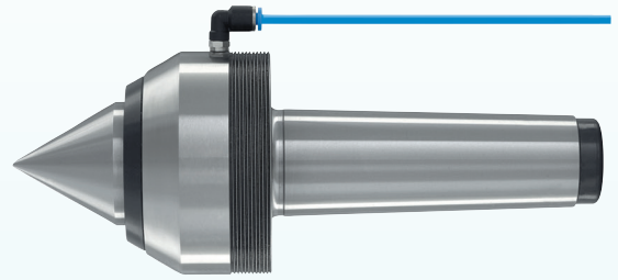
mit Sperrluftanschluss
