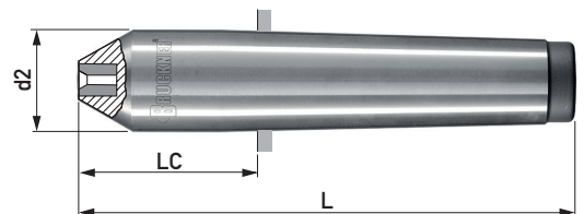
Form B *Rundheitstoleranz \square \leq 1 \mu\text{m}
