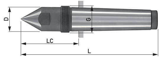
Form 255 ähnlich DIN 807 und verlängert, 60°
