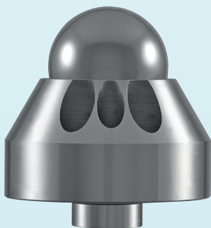
offene Zentrierbohrung
