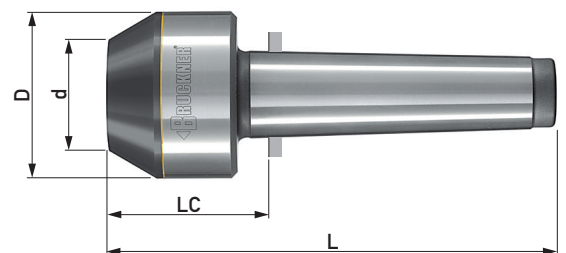
Form R großer Hartmetallring bis \varnothing 100 \text{ mm}
