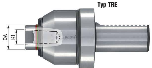
Zentriereinsätze für Typ TRE Seite 43
