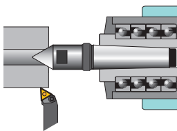
Form 255 für kleine und große Zentren
