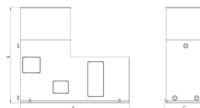
BKD 520 (mit Ansaug- und Ausblas Kulissenschalldämpfer)
