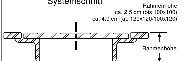
Systemschnitt
