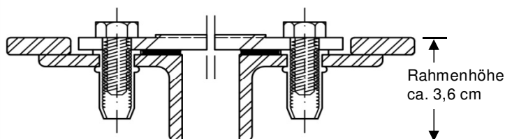
Systemschnitt Sechskantschraube
