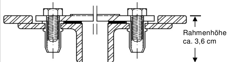
Systemschnitt Sechskantschraube
