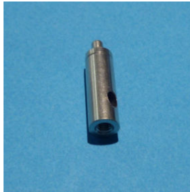
Drahtseilhalter M5 messing-vernickelt, Gewinde: M5 für Drahtseile 1,0 bis 1,5 mm \varnothing seitlicher Seilausgang Art-Nr. 10-105001-03 Verpackungseinheit: 100 Stück 245,00 € per 100 Stück
