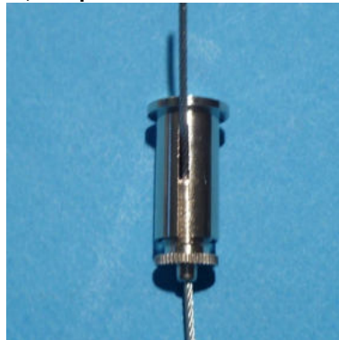
Deckenbefestiger mit Schlitz und Bohrung M6 mit Drahtseilhalter für Seile 1,0 bis 1,5 mm ø Art-Nr. 10-125001-03 Verpackungseinheit: 10 Stück 2,96 € per Stück
