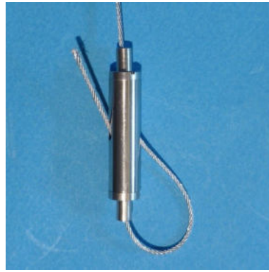
Drahtseilhalter zur Schlaufenbildung, vernickelt für Drahtseile 1,0 bis 1,6 mm ø zweifacher seitlicher Seilausgang Art-Nr. 10-135001-03 Verpackungseinheit: 10 Stück 3,60 € per Stück
