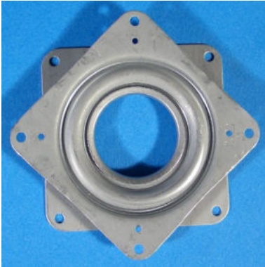
Kugellager 75 x 75 x 8 mm aus verzinktem Stahlblech Innen-ø: 33 mm max. Auflage: bis 45 cm ø max. Belastung: 90 kg Art-Nr. 05-075075-04 3,95 € per Stück
