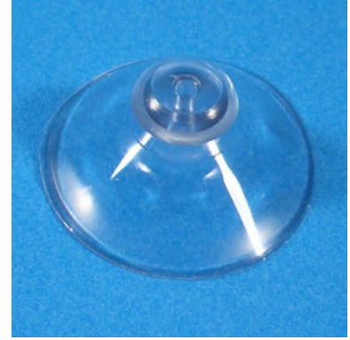
Haftsauger 40 mm ø , transparent mit Knopf-ø 15 mm, Hals-ø 10 mm Art-Nr. 01-341200-11 Verpackungseinheit: 100 Stück 19,95 € per 100 Stück
