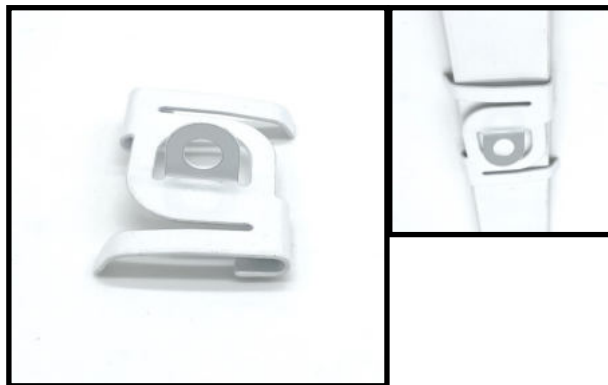
Decken-Clip, weiß 38 x 28 mm, Öse: 5 mm ø Art-Nr. 01-118000-05 Verpackungseinheit: 100 Stück 120,00 € per 100 Stück
