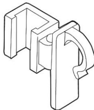
Aufhängehaken 2-teilig zum einhängen von Rahmen an Drahtgittern bis max. 12 mm Ø, grau Art-Nr. 08-100136-15 Verpackungseinheit: 10 Paar 1,16 € per Paar
