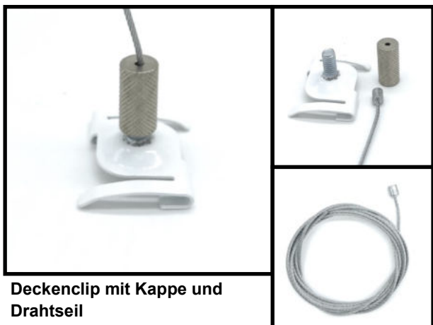
Decken-Clip, weiß 38 x 28 mm, mit Gewinde M6 x 10 mm Art-Nr. 01-600044-05 Verpackungseinheit: 100 Stück 150,00 € per 100 Stück
