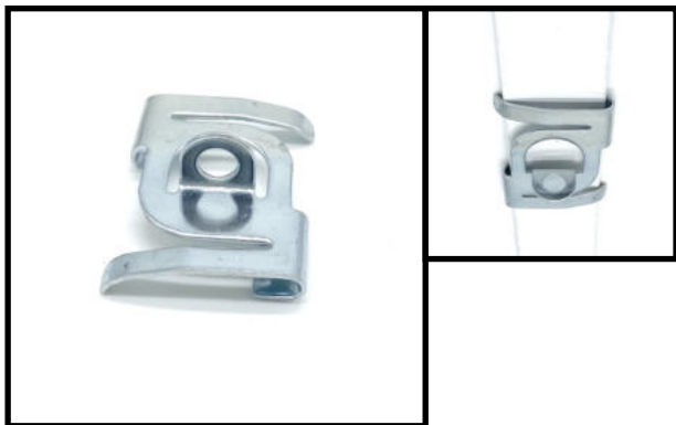
Decken-Clip, verzinkt 38 x 28 mm, Öse: 5 mm ø Art-Nr. 01-118000-01 Verpackungseinheit: 100 Stück 120,00 € per 100 Stück
