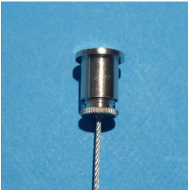
Deckenbefestiger, kurz mit Bohrung M6 + Schraubkappe für Drahtseile einseitig mit Nippel Art-Nr. 10-120001-03 Verpackungseinheit: 10 Stück 2,30 € per Stück
