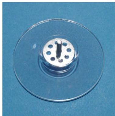
Haftsauger 75 mm ø , transparent mit Gewinde M4 x 14 mm lang Art-Nr. 01-370750-11 Verpackungseinheit: 100 Stück 213,00 € per 100 Stück
