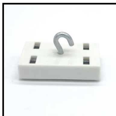
Deckenmagnet weiß, mit Haken kunststoffummantelt Abm.: 53 x 27 x 28 mm Haftkraft: 15 kg Art-Nr. 03-510040-05 Verpackungseinheit: 60 Stück
