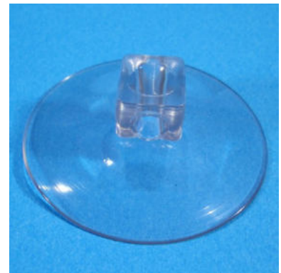
Haftsauger 60 mm ø , transparent mit Querloch 6 mm ø Art-Nr. 01-380600-11 Verpackungseinheit: 100 Stück 47,00 € per 100 Stück
