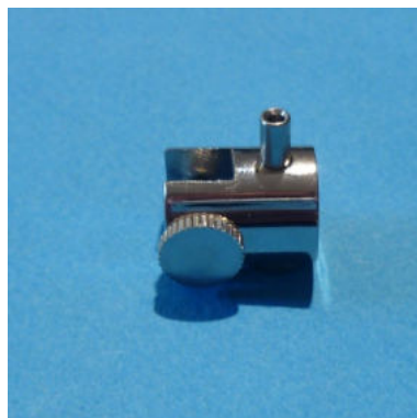
Drahtseilhalter, links vernickelt für Displays bis 6,5 mm Stärke Rändelschraube links für Drahtseile 1,0 bis 1,5 mm ø Art-Nr. 10-131001-03 Verpackungseinheit: 10 Stück 4,00 € per Stück
