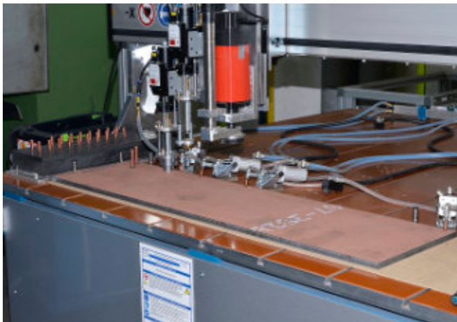
AUTOMATISCHE BOLZENSCHWEIßANLAGE Arbeitsbereich von XY – 1050 mm x 1500 mm ermöglicht das präzise, vollautomatische Aufschiessen von Bolzen und Stiften von Ø 3 - 10 mm und 40 mm Länge
