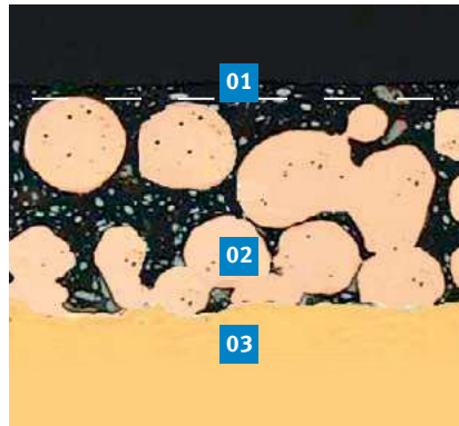
Abb. 16: Schichtsystem P11
