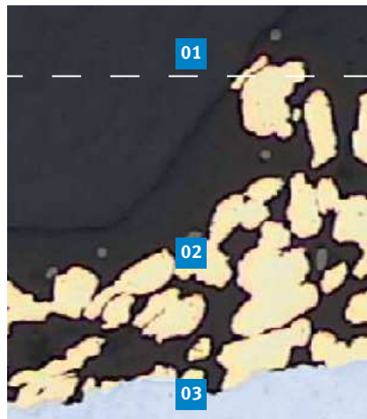
Abb. 22: Schichtsystem
