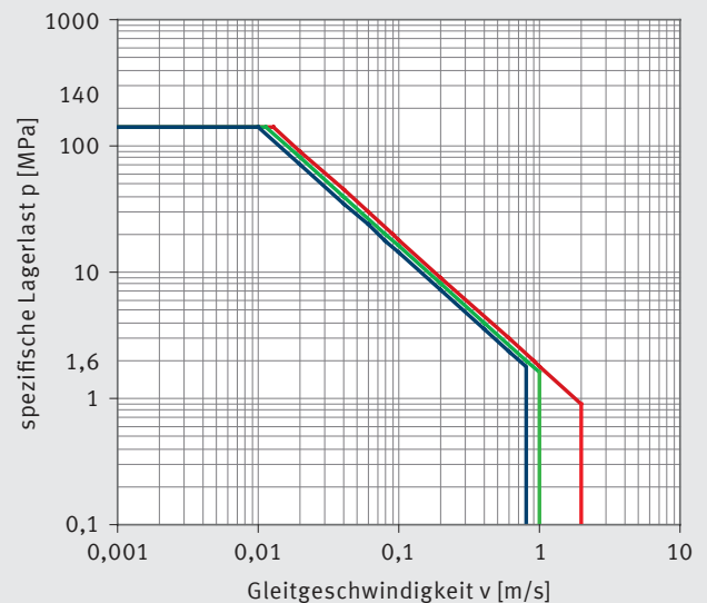
Abb. 10: pv-Wert [MPa · m/s], Grenzkurve (Werte gültig bei Raumtemperatur)
